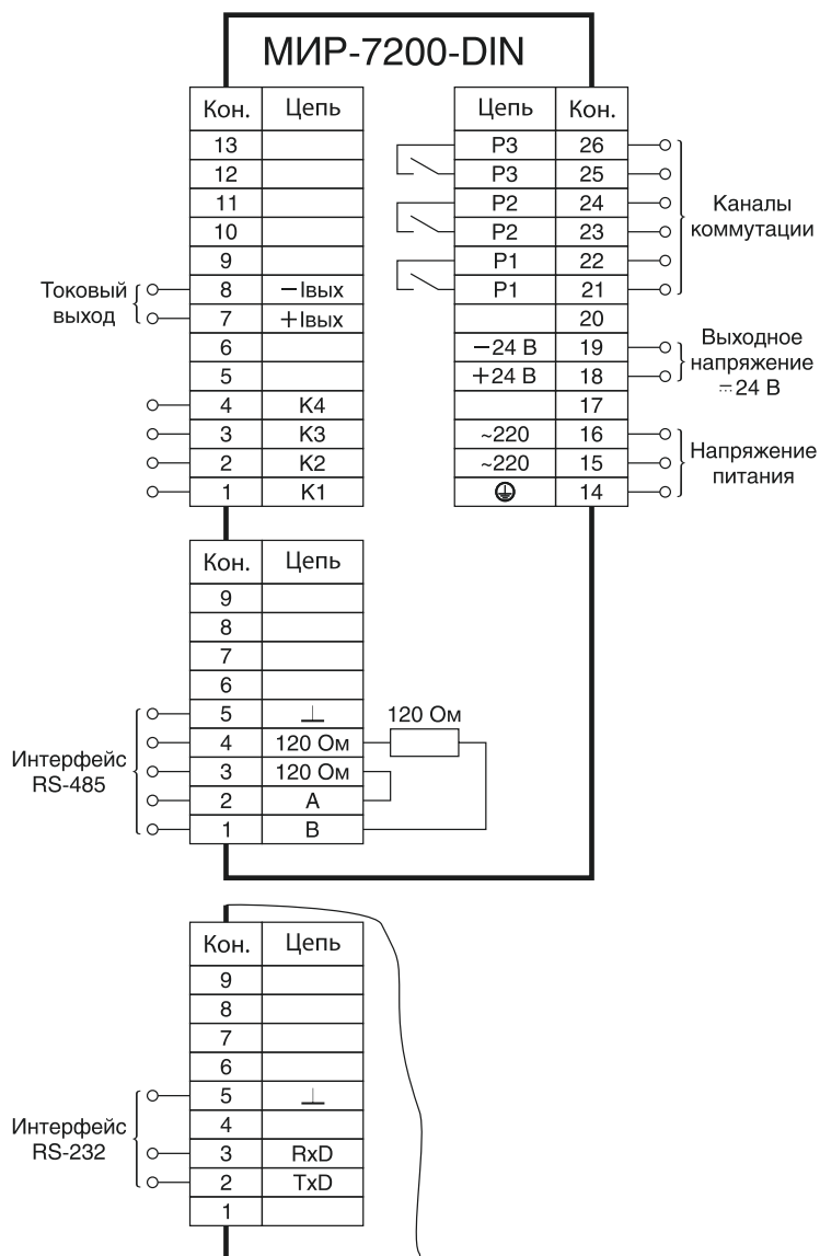
Рисунок Б.1 — Схема подключения к регулятору исполнения DIN
