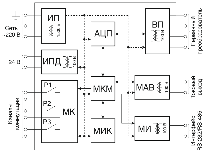
Рисунок 1 — Функциональная схема регуляторов в исполнении DIN и 01
