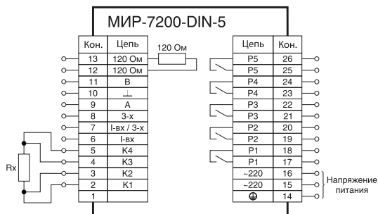
Рисунок В.7 — Схема подключения регулятора исполнения DIN с пятью каналами коммутации при определении приведенной погрешности в режимах измерения сопротивления, сигналов от термопреобразователей сопротивления
