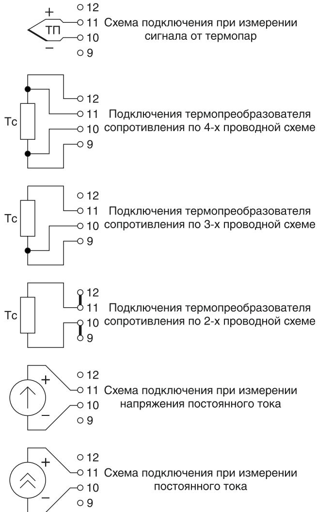
Рисунок Б.4 — Схемы подключений термопар, термопреобразователей сопротивления по 4-х, 3-х и 2-х проводным схемам, подключения при измерении напряжения постоянного тока и силы постоянного тока к регулятору исполнения 01
