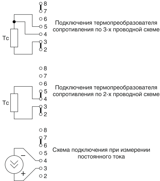
Рисунок Б.9 — Схемы подключений термопреобразователей сопротивления по 2-х и 3-х проводным схемам, подключение при измерении силы постоянного тока к регулятору исполнения DIN с пятью каналами коммутации
