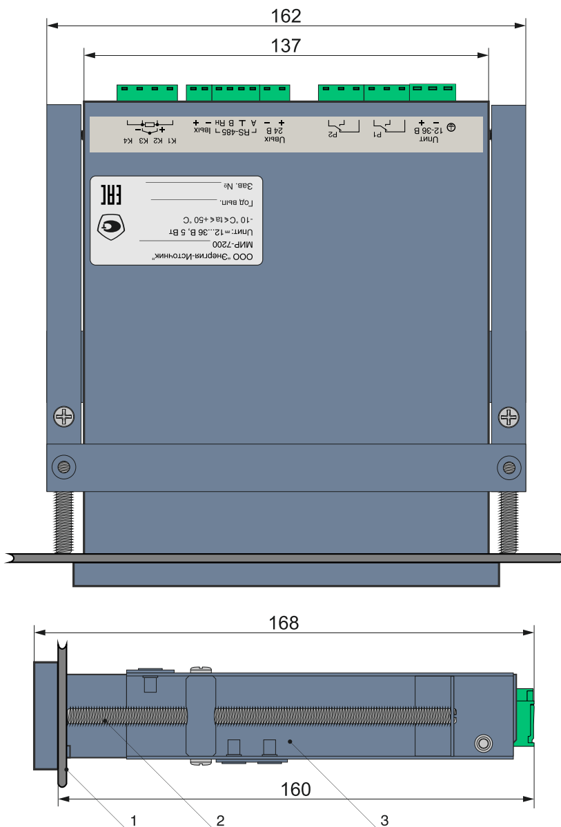
Рисунок А.7 — Внешний вид и габаритные размеры регулятора исполнения 03
