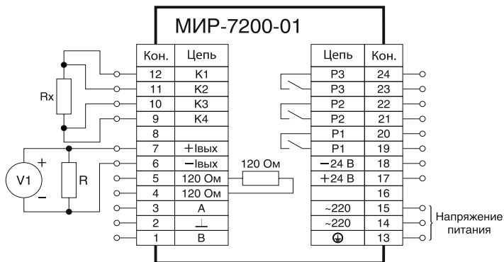
Рисунок В.5 — Схема подключения регулятора исполнения DIN при определении приведенной погрешности в режимах измерения сопротивления, сигналов от термопреобразователей сопротивления
