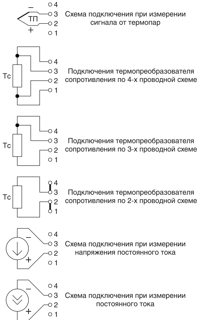
Рисунок Б.2 — Схемы подключений термопар, термопреобразователей сопротивления по 4-х, 3-х и 2-х проводным схемам, подключения при измерении напряжения постоянного тока и силы постоянного тока к регулятору исполнения DIN
