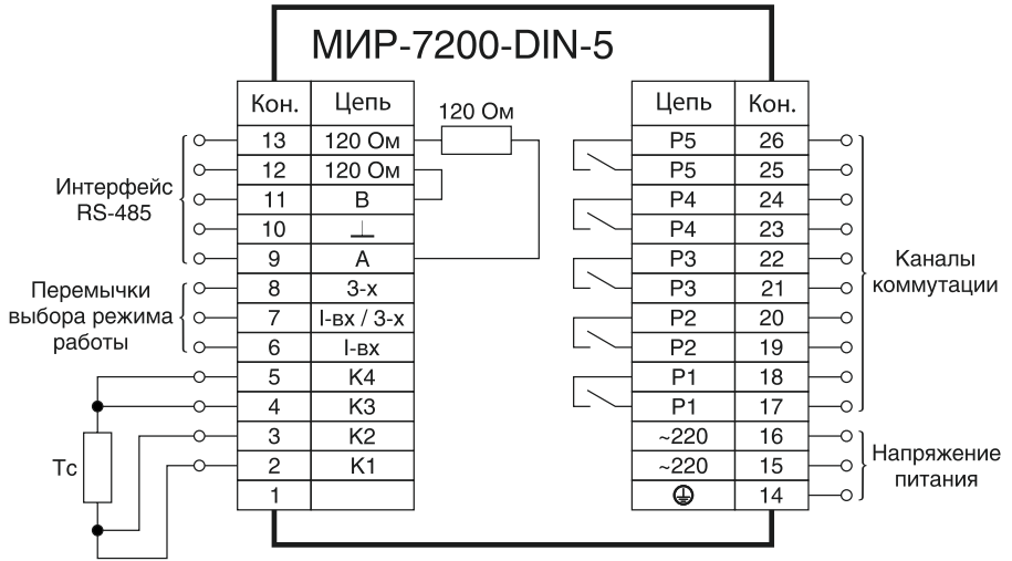
Рисунок Б.8 — Схема подключения к регулятору исполнения DIN с пятью каналами коммутации термопреобразователя сопротивления по четырехпроводной схеме
