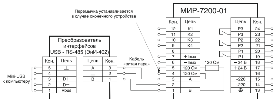
Рисунок Б.11 — Схема подключения регуляторов с интерфейсом RS-485 к компьютеру
