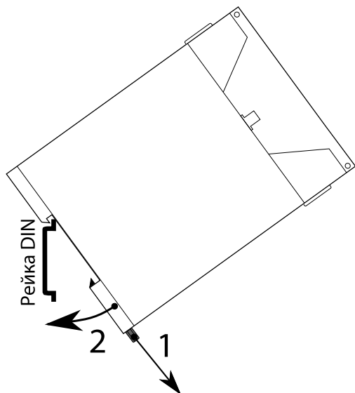
Рисунок 4 — Монтаж регулятора исполнения DIN на DIN-рейку
