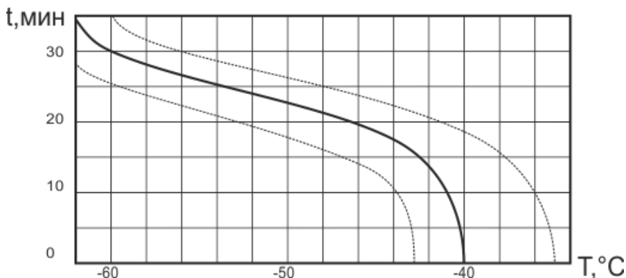
Рисунок Г.1 — Время включения регулятора после самопрогрева при температуре ниже минус 35 °С
