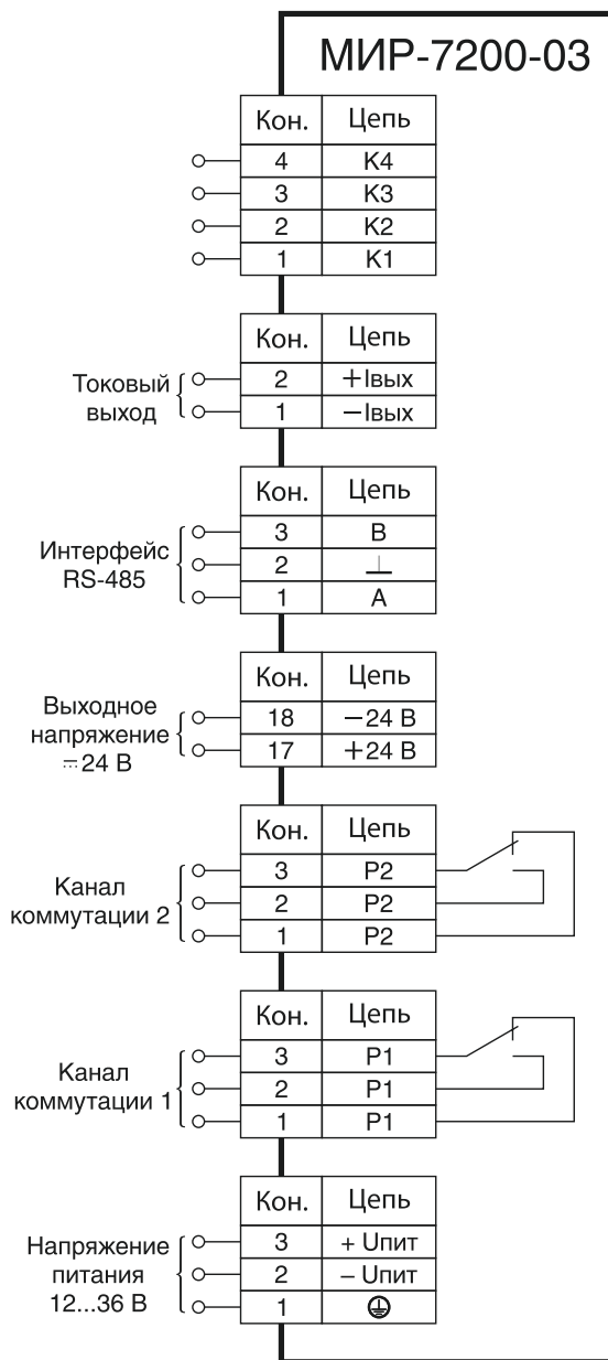
Рисунок Б.6 — Схема подключения к регулятору исполнения 03
