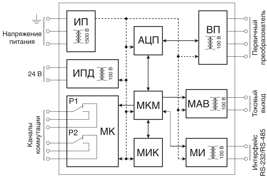
Рисунок 2 — Функциональная схема регулятора в исполнении 02 и 03
