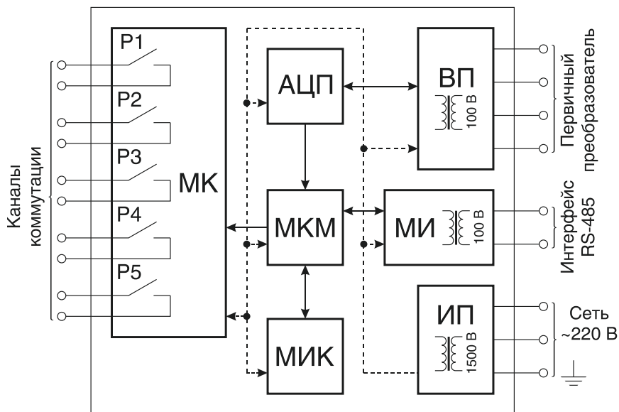
Рисунок 3 — Функциональная схема регулятора в исполнении DIN с пятью каналами коммутации
