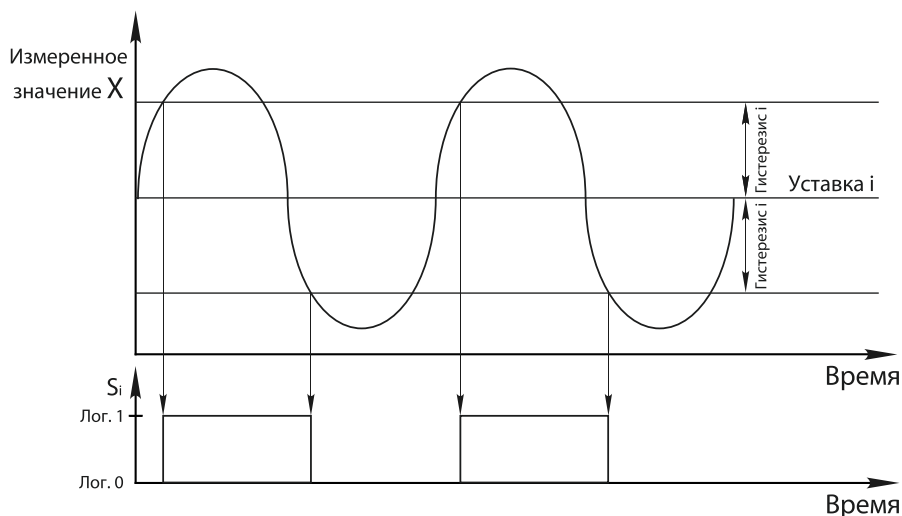
Рисунок 11 — Логика работы пороговых устройств
