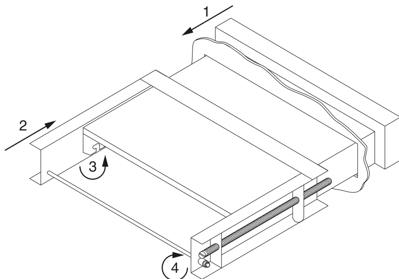
Рисунок 6 — Монтаж регулятора исполнения 01 в щит
