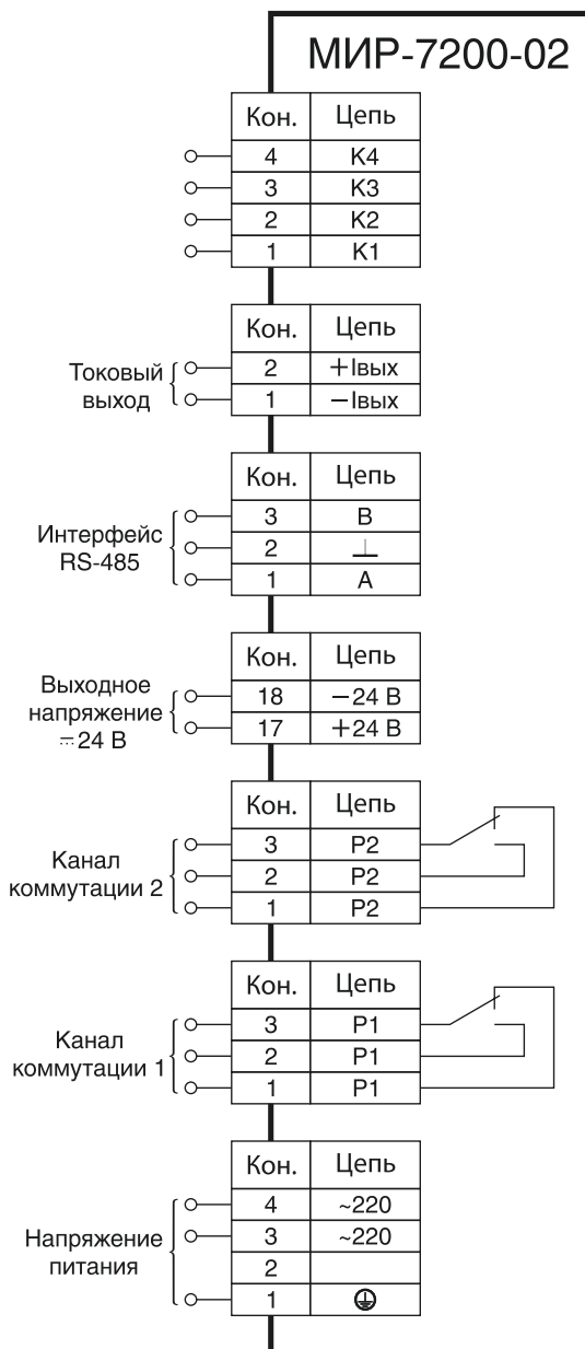
Рисунок Б.5 — Схема подключения к регулятору исполнения 02
