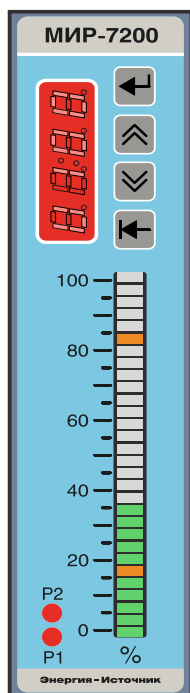
Рисунок А.8 — Внешний вид регулятора исполнения 03 при установке в вертикальной ориентации
