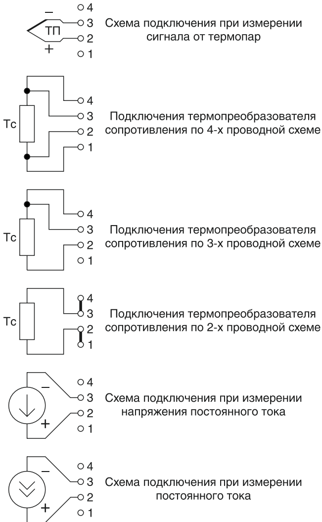
Рисунок Б.7 — Схемы подключений термопар, термопреобразователей сопротивления по 4-х, 3-х и 2-х проводным схемам, подключения при измерении напряжения постоянного тока и силы постоянного тока к регулятору исполнения 02 и 03
