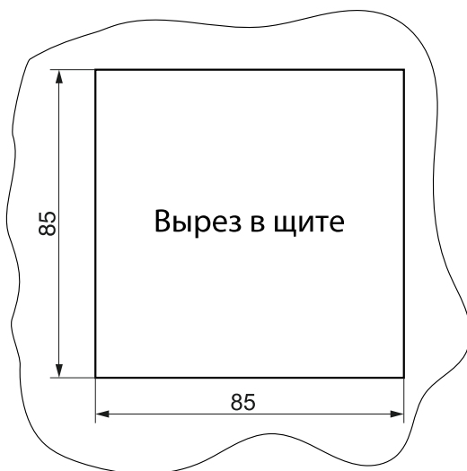
Рисунок А.9 — Разметка отверстия в щите для установки регулятора исполнения 01
