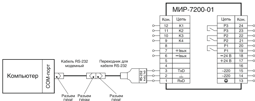
Рисунок Б.10 — Схема подключения регуляторов с интерфейсом RS-232 к компьютеру
