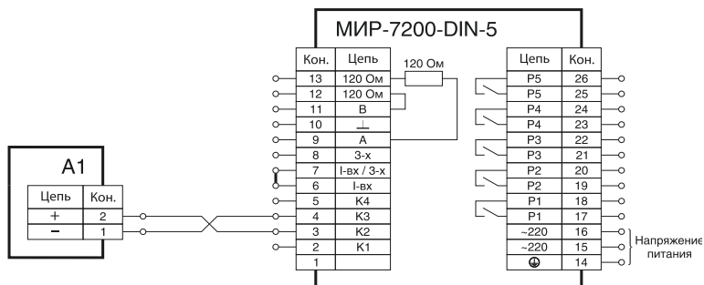
Рисунок В.3 — Схема подключения регулятора исполнения DIN с пятью каналами коммутации при определении приведенной погрешности в режиме измерения тока
