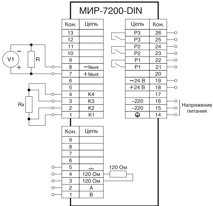
Рисунок В.5 — Схема подключения регулятора исполнения DIN при определении приведенной погрешности в режимах измерения сопротивления, сигналов от термопреобразователей сопротивления
