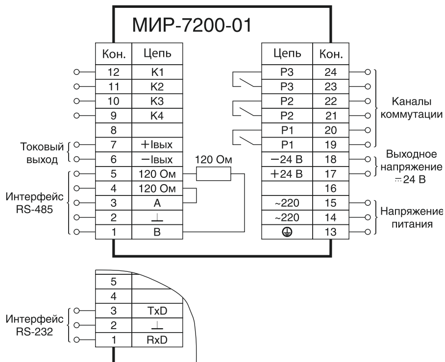
Рисунок Б.3 — Схема подключения к регулятору исполнения 01
