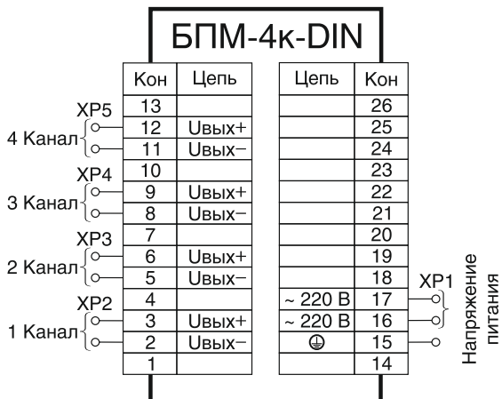
Рисунок Б.9 — Схема подключения блоков БПМ-4к (исполнение DIN)
