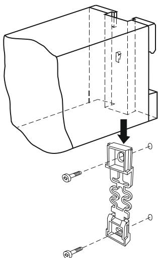
Рисунок 2 — Монтаж блоков на DIN-рейку
