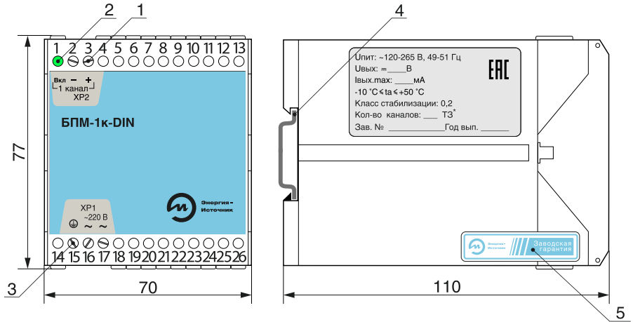
Рисунок А.9 — Габаритные размеры блоков БПМ-1к (120, 250, 500 мА) (исполнение DIN)
