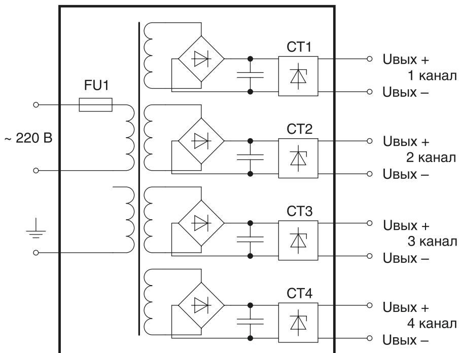
Рисунок 1 — Функциональная схема блоков
