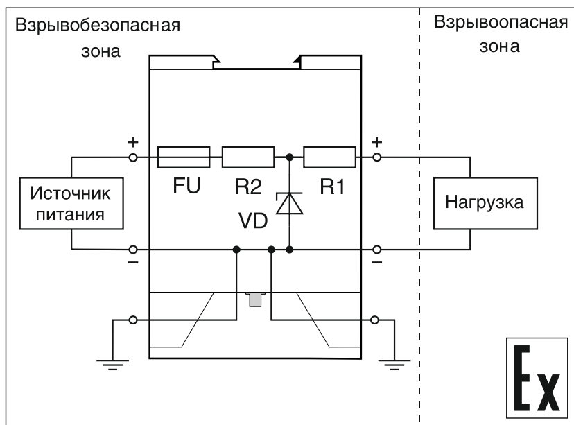
Рисунок 1 — Функциональная схема
